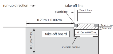
Rys. (a2) TR29 – Belka do odbicia z wkładką z plasteliną
